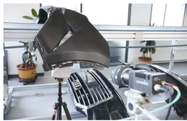
易启科技开发的汽车行业大幅面曲面智能检测系统
